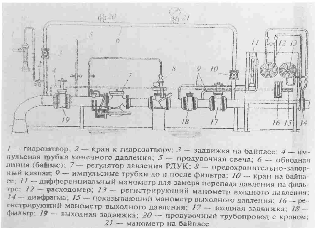
Рис. 1 Газорегуляторный пункт
